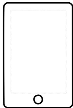
Ecranul
