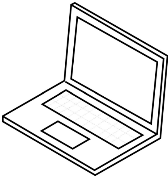
Tastatura
