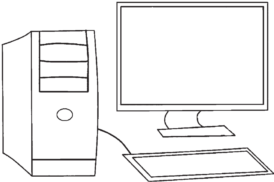
Unitatea centrală
